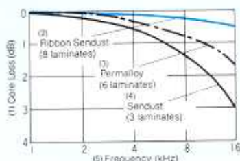
(1) Pérdidas en el núcleo (dB) (2) Ribbon Sendust (8 láminas) (3) Permalloy (5 láminas) (4) Sendust (3 láminas) (5) Frecuencia (KHz)
