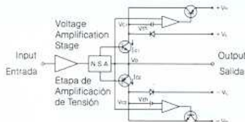
N.S.A. = Non-Switching Amp N.S.A. = Amplificador Non-Switching
