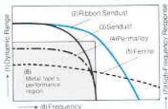
(1) Gama dinámica (2) Ribbon Sendust (3) Sendust (4) Permalloy (5) Ferrita (6) Zona de rodamiento de las cintas de metal (7) Respuesta de alta frecuencia (8) Frecuencia
